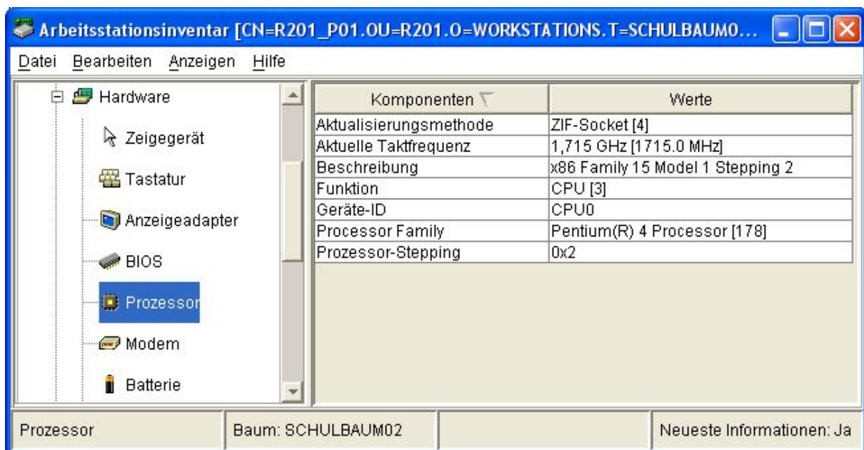
Bild 1: Abfrage der Inventardaten einer Arbeitsstation
